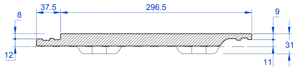
Schnitt A-A
